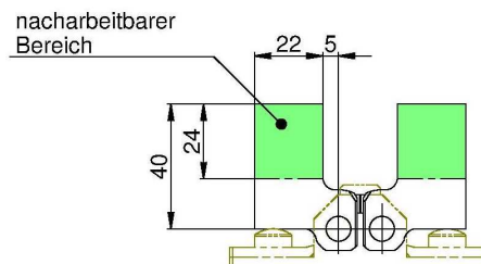
Abbildung 4: BG nacharbeitbarer Spannschraube
