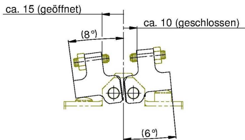
Abbildung 3: BG Spannschraube (Standard)
